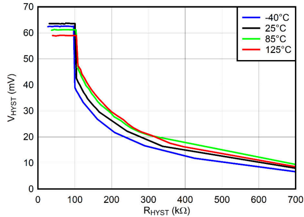
图 7-4. V HYST (mV) vs R HYST (kΩ), V CC = 3.3V
