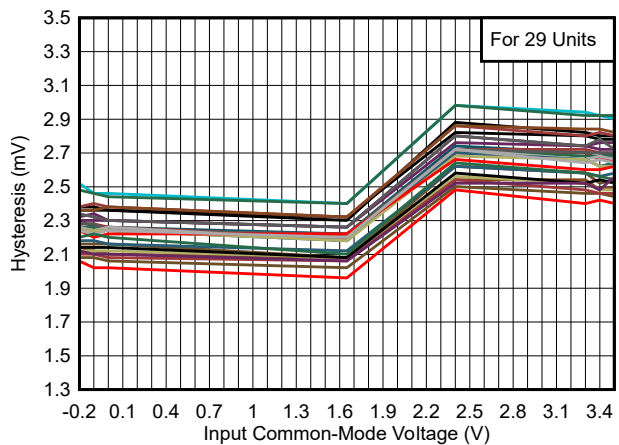
图 5-4. 迟滞与共模电压间的关系, 3.3V
