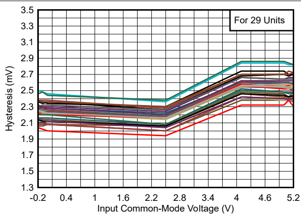
图 5-6. 迟滞与共模电压间的关系, 5V
