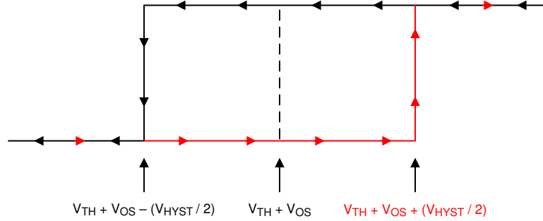
图 6-1. 迟滞传递曲线
