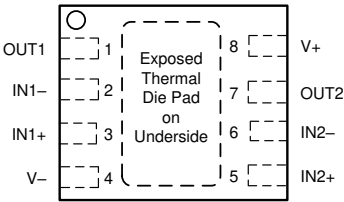
DSOG 封装 8 引脚 WSON (带有外露散热焊盘) 顶视图
