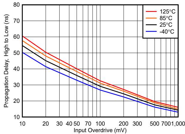
图 5-27. 在 1.8V 时高电平到低电平的传播延迟与过驱间的关系
