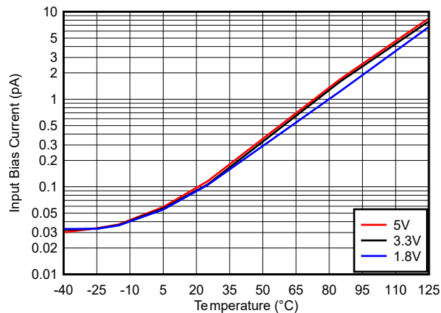
图 5-17. 输入偏置电流与 温度间的关系
