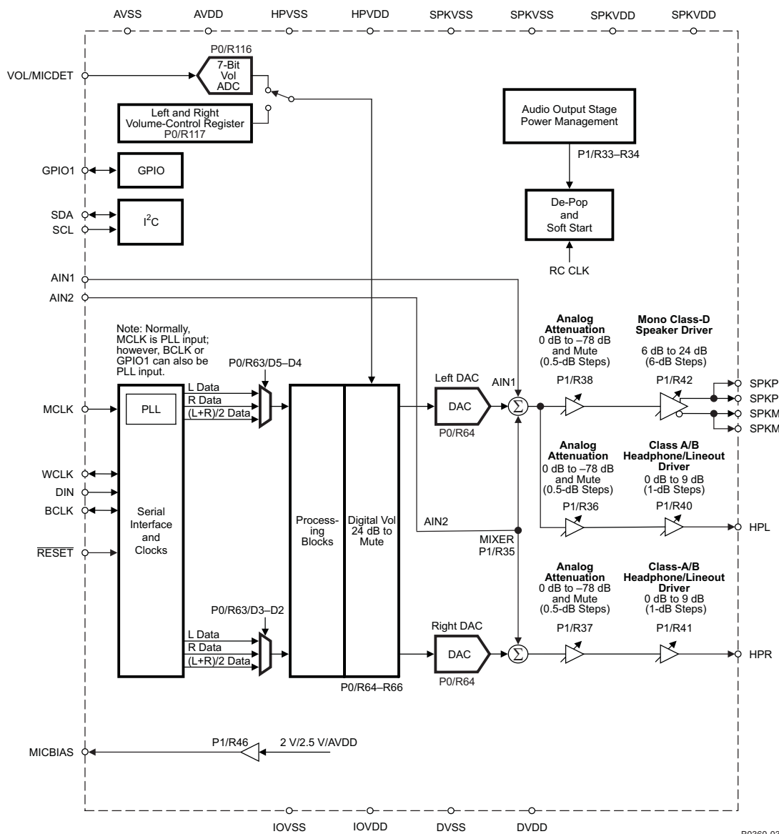
图 1-1. 功能方框图
