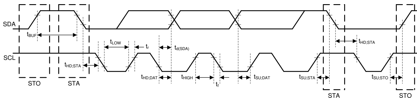
图 7-1. I 2 C Interface Timing Diagram
