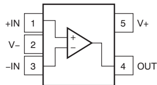
DCK 封装: TLV314 5 引脚 SC70 顶视图
