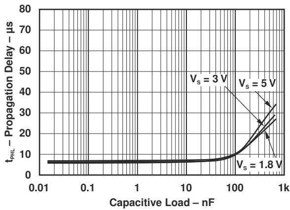
图 7-7. 传播延迟时间 ( t_{PHL} ) 与容性负载间的关系
