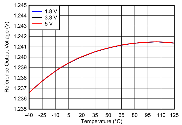
图 8-16. 基准电压与温度间的关系
