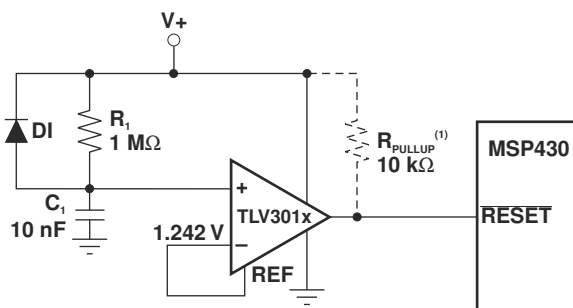
图 10-5. TLV3012 配置为 MSP430™ 微控制器的上电复位电路
