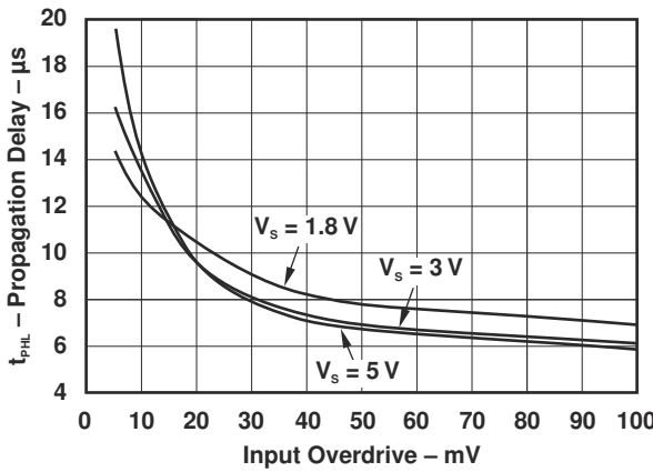
图 7-9. 传播延迟时间 ( t_{PHL} ) 与输入过驱间的关系
