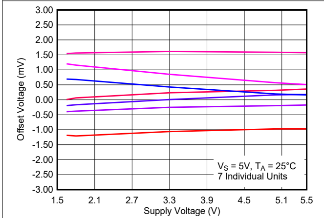
图 8-33. 失调电压与电源电压间的关系, 25°C
