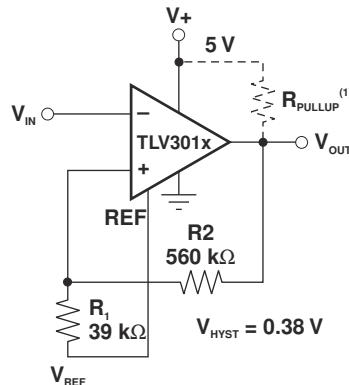
图 10-2. 添加迟滞
