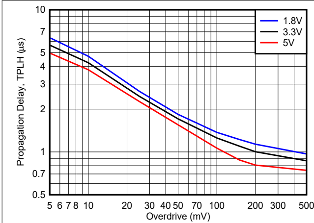
图 8-13. 从低电平到高电平传播延迟时间与过驱间的关系
