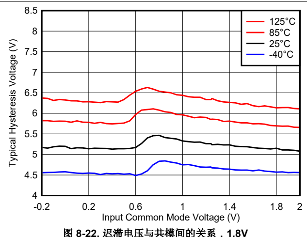
图 8-22. 迟滞电压与共模间的关系, 1.8\text{V}
