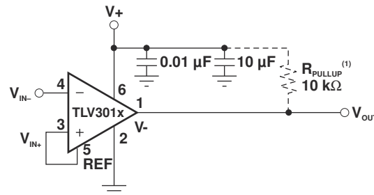
图 10-1. 基本连接
