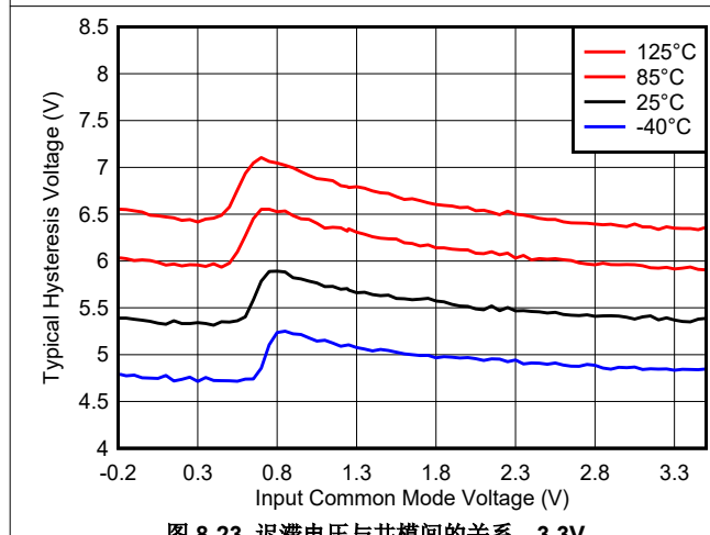
图 8-23. 迟滞电压与共模间的关系, 3.3\text{V}
