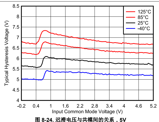
图 8-24. 迟滞电压与共模间的关系, 5\text{V}
