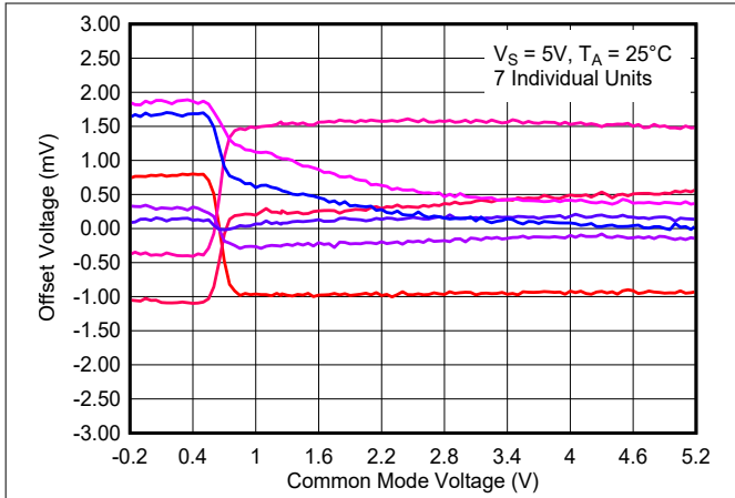
图 8-31. 失调电压与共模电压间的关系, 5V
