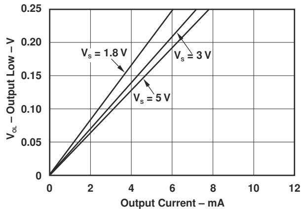
图 6-4. OUTPUT LOW vs OUTPUT CURRENT
