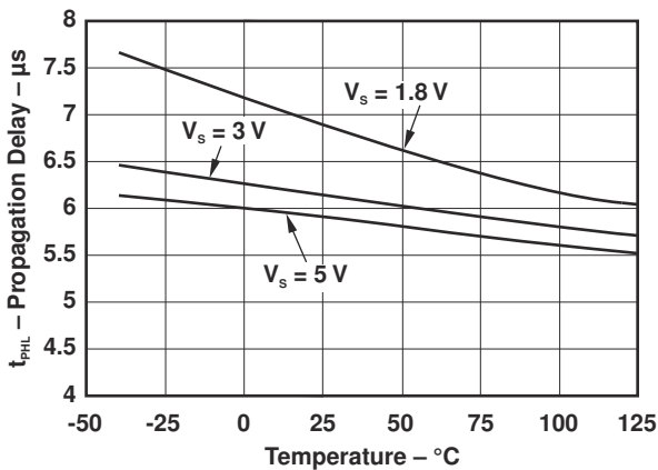
图 7-11. 传播延迟时间 ( t_{\text{PHL}} ) 与温度间的关系
