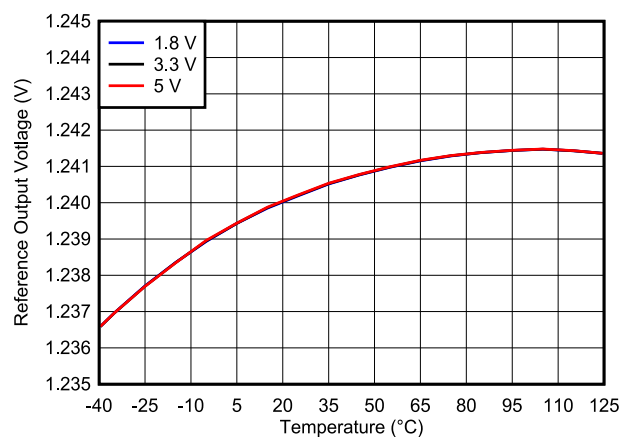
TLV3012B 基准电压与温度间的关系
