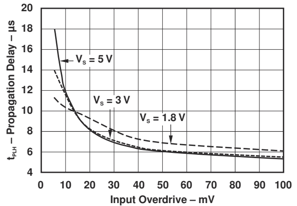
图 7-8. 传播延迟时间 ( t_{\text{PLH}} ) 与输入过驱间的关系
