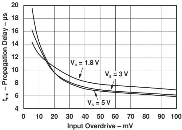
图 7-9. 传播延迟时间 ( t_{\text{PHL}} ) 与输入过驱间的关系
