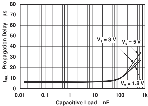
图 7-7. 传播延迟时间 ( t_{\text{PHL}} ) 与容性负载间的关系
