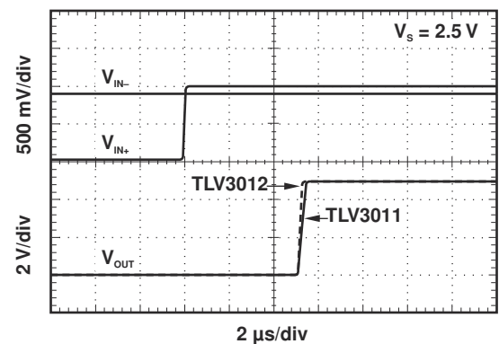
图 7-12. 传播延迟时间 ( t_{\text{PLH}} )
