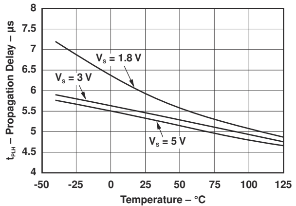
图 7-10. 传播延迟时间 ( t_{\text{PLH}} ) 与温度间的关系
