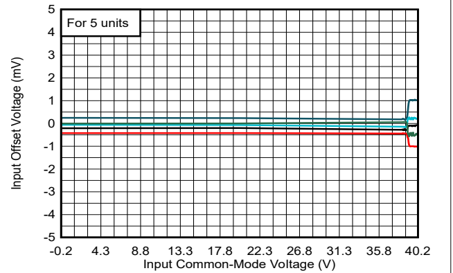
图 5-4. 失调电压与共模电压间的关系, 40V
