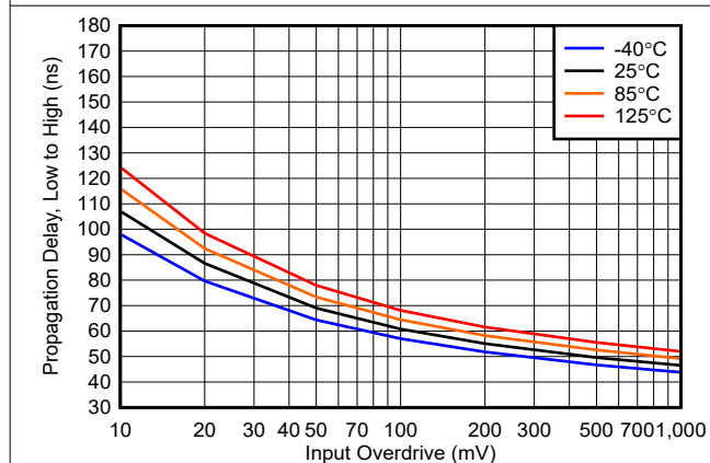
图 5-23. 传播延迟 (低电平到高电平) 与输入过驱间的关系, 40V
