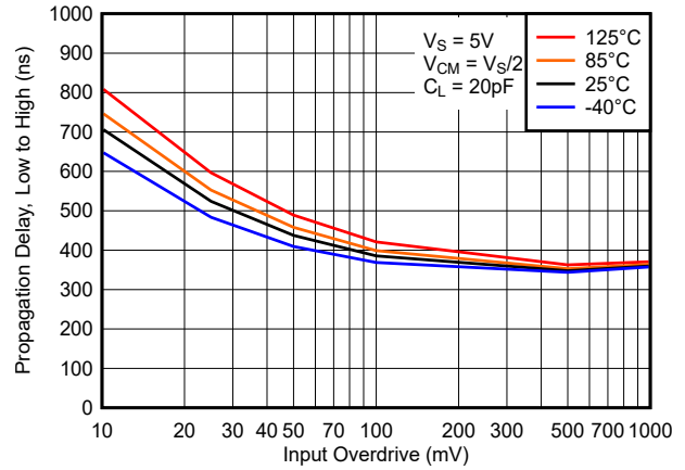
图 6-14. 传播延迟, 从低电平到高电平, 5V
