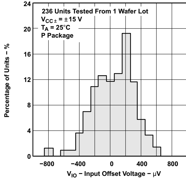
图 5-1. TLE2141 输入失调电压的分布
