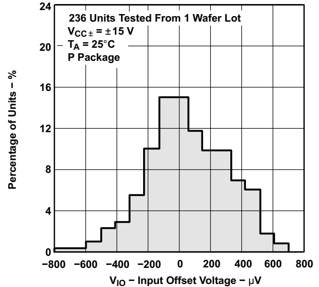
图 5-2. TLE2142 输入失调电压的分布
