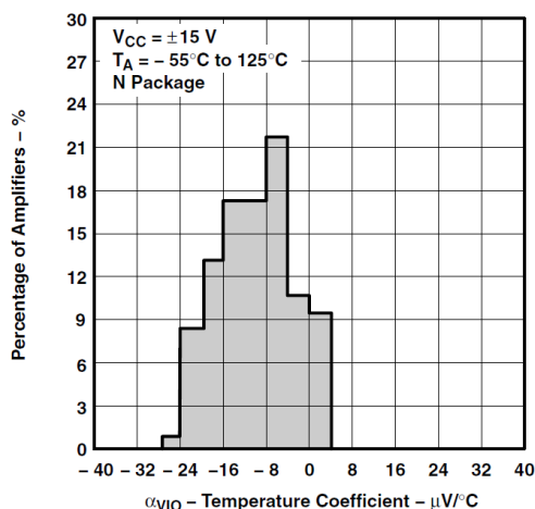
图 6-6. TLE2074 输入失调电压温度系数的分布
