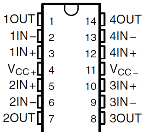
图 5-4. TLE2074 和 TLE2074A J、N 或 W 封装 (顶视图)
