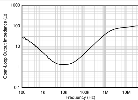
图 6-15. 开环输出阻抗与频率间的关系
