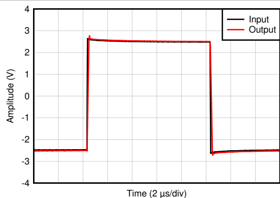
图 6-13. 小信号脉冲响应
