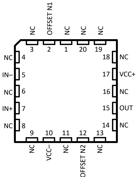
图 5-6. TLE2071M 和 TLE2071AM FK 封装 (顶视图)
