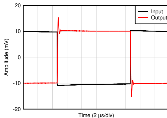
图 6-14. 小信号脉冲响应
