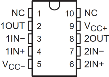
图 4-8. TLE2062 和 TLE2062A U 封装 ( 顶视图 )
