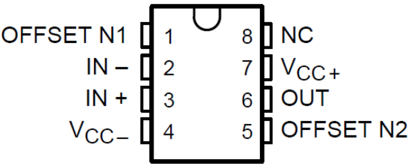
图 4-1. TLE2061、TLE2061A 和 TLE2061B D、DB、JG、P 或 PW 封装 ( 顶视图 )
