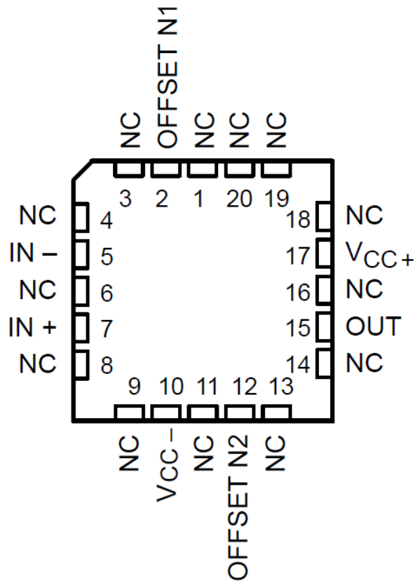
图 4-4. TLE2061M、TLE2061AM 和 TLE2061BM FK 封装 (顶视图)
