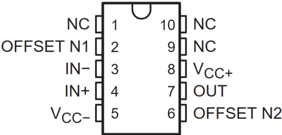
图 4-7. TLE2061 和 TLE2061A U 封装 ( 顶视图 )
