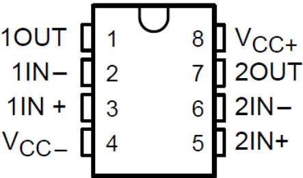
图 4-2. TLE2062、TLE2062A 和 TLE2062B D、JG 或 P 封装 ( 顶视图 )
