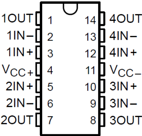
图 4-3. TLE2064、TLE2064A 和 TLE2064B D、J、N 或 W 封装 ( 顶视图 )
