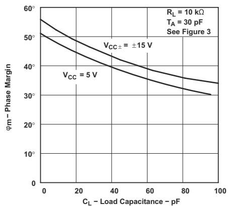
图 6-49. TLE2021 相位裕度与负载电容间的关系
