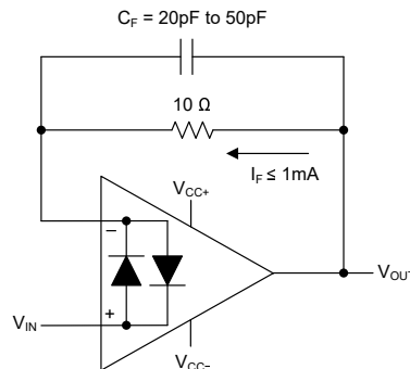
图 7-1. 电压输出器
