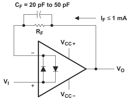
图 8-1. 电压输出器
