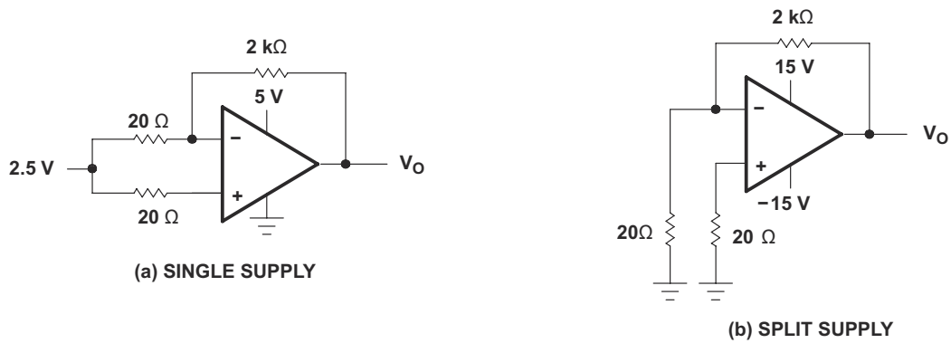
图 6-2. 噪声电压测试电路
