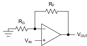
图 7-3. 原理图表示
