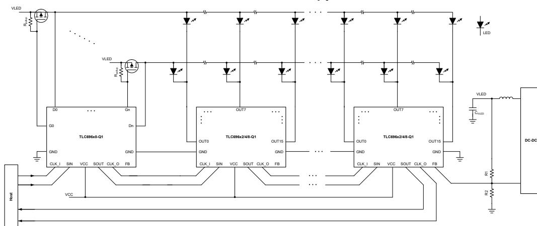
简化原理图
