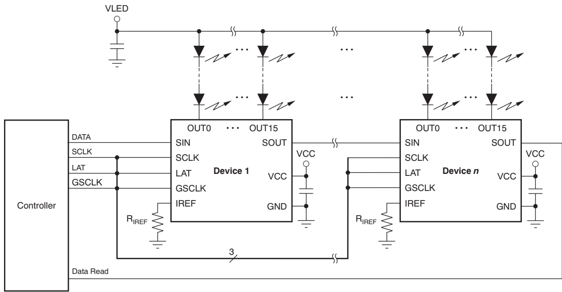
典型应用电路（多菊花链 TLC59482）
