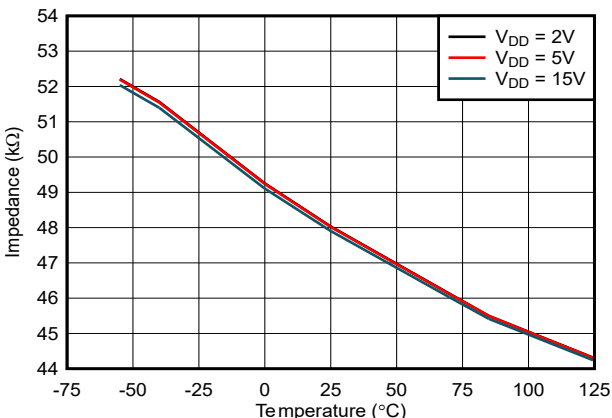
图 5-4. 控制阻抗与温度间的关系
