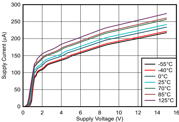
图 5-3. 电源电流与电源电压间的关系
