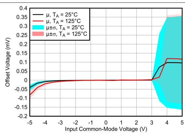
图 7-4. 失调电压与输入共模电压间的关系
