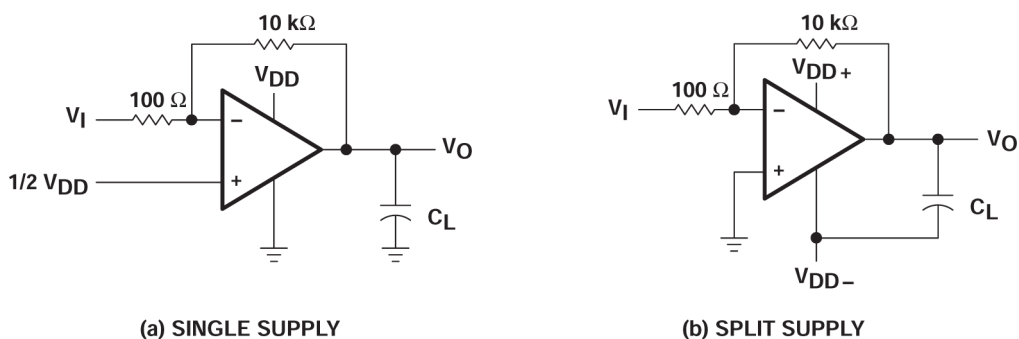
图 6-3. 100 倍增益反相放大器
