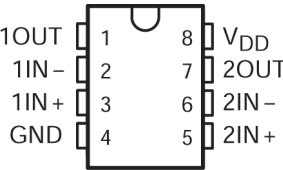
图 4-1. D ( 8 引脚 SOIC )、P ( 8 引脚 PDIP )、PS ( 8 引脚 SOP ) 或 PW ( 8 引脚 TSSOP ) 封装 ( 俯视图 )
