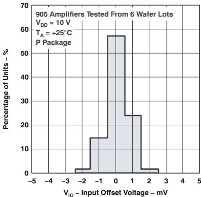
图 5-2. TLC27L1 输入 偏移电压的分布
