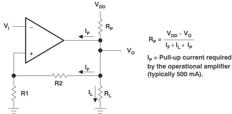
图 7-9. 使用电阻式上拉电阻器来提高 V_{OH}
