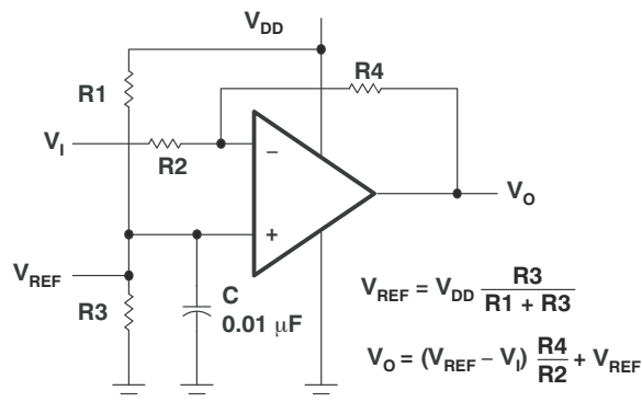
图 7-1. 具有电压基准的反相放大器
