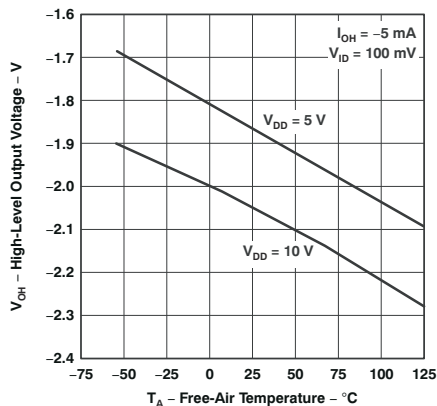
图 5-8. 高电平输出电压 与 自然通风温度间的关系
