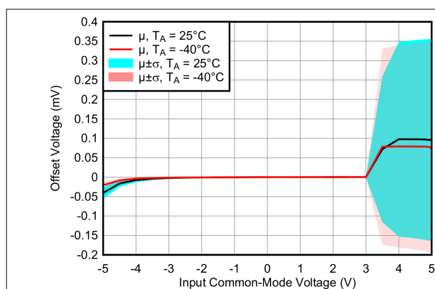
图 7-3. 偏移电压与输入共模电压间的关系
