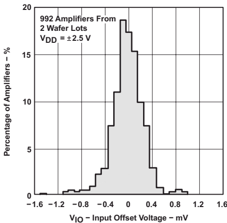
图 6-3. Distribution of TLC2274-Q1 Input Offset Voltage
