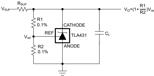
图 9-1. 并联稳压器原理图
