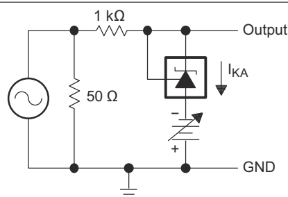
图 6-8. 基准阻抗测试电路
