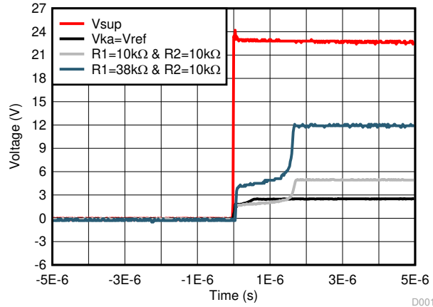
图 9-2. TLA431 启动响应
