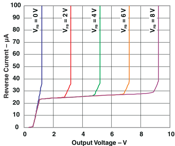
图 5-5. 反向特性
