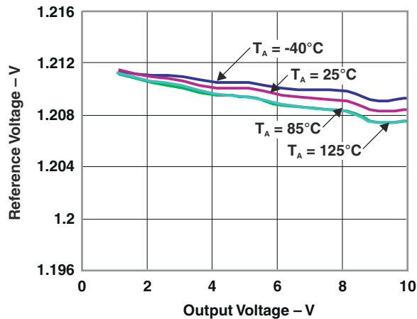
图 5-9. 基准电压与输出电压间的关系
