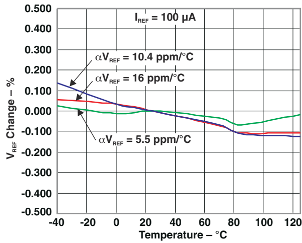
图 5-1. 不同平均温度系数的温度漂移
