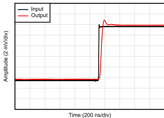
图 5-27. 正过载恢复
