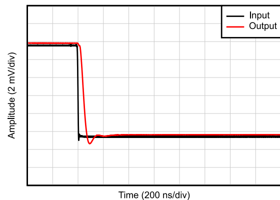
图 5-28. 负过载恢复
