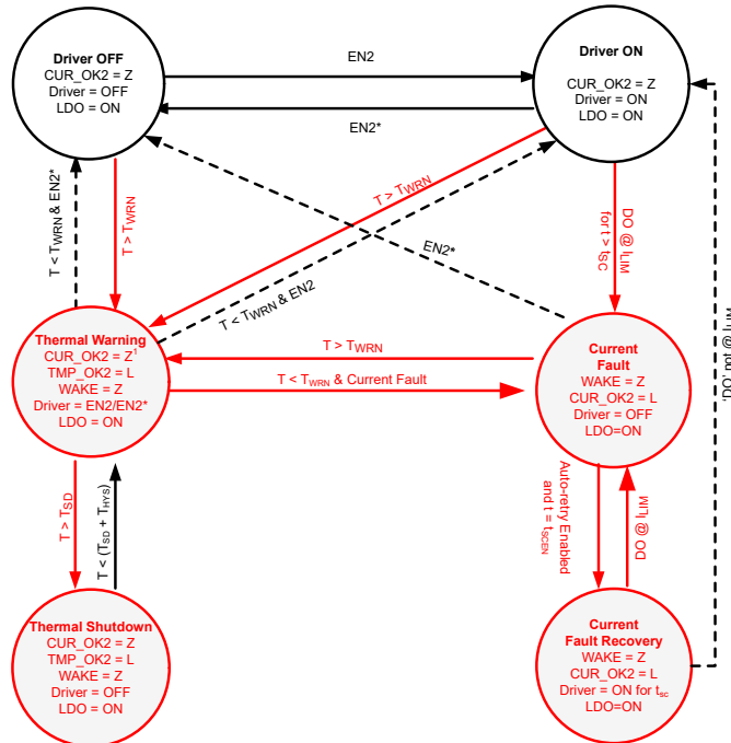
图 7-3. DO 驱动器状态图
