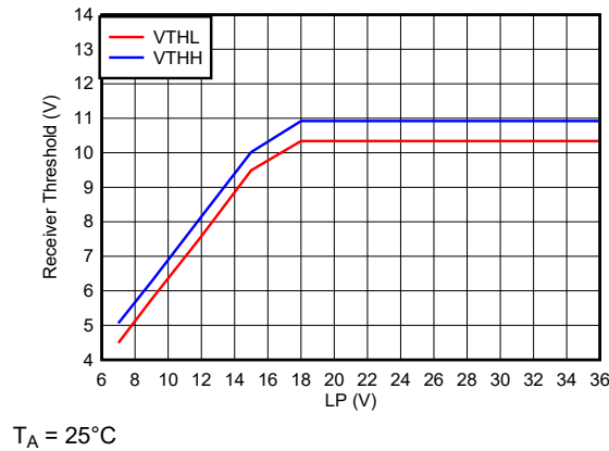
图 5-5. CQ、DI 接收器阈值边界
