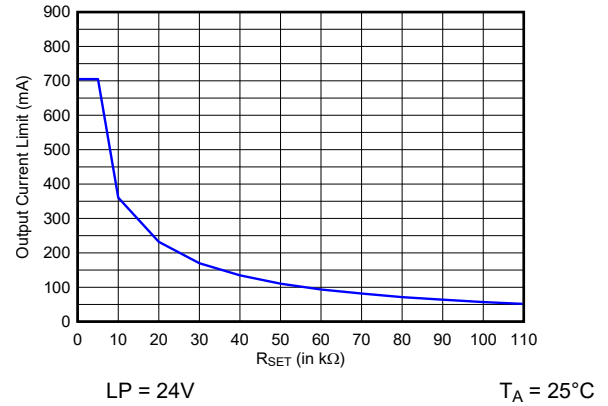
图 5-4. CQ、DO 电流限值与 0-5k \Omega 范围内的 R SETx 1
