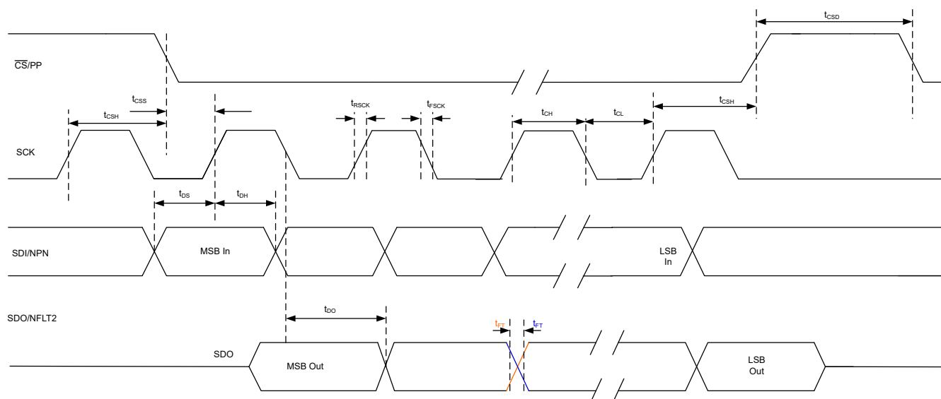
图 6-8. SPI 读/写时序特性
