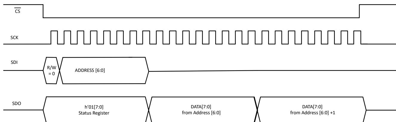
图 7-7. SPI 读取 (突发模式)
