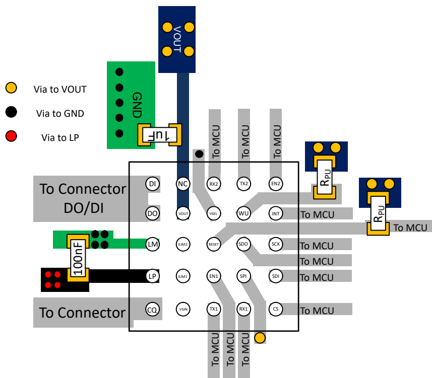
图 8-9. DSBGA 布局示例 (显示的是 SPI 模式)
