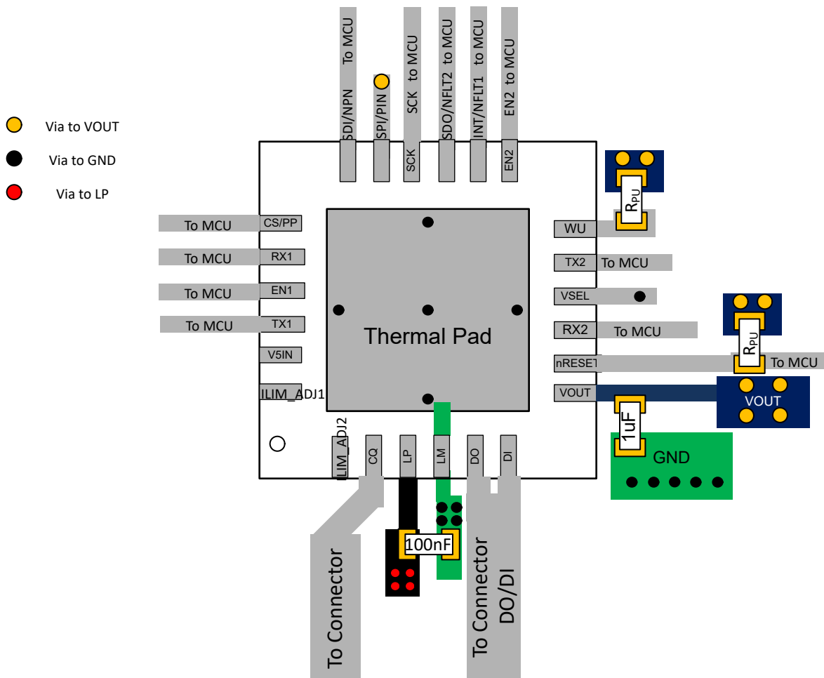
图 8-8. QFN 布局示例 ( 显示的是 SPI 模式 )
