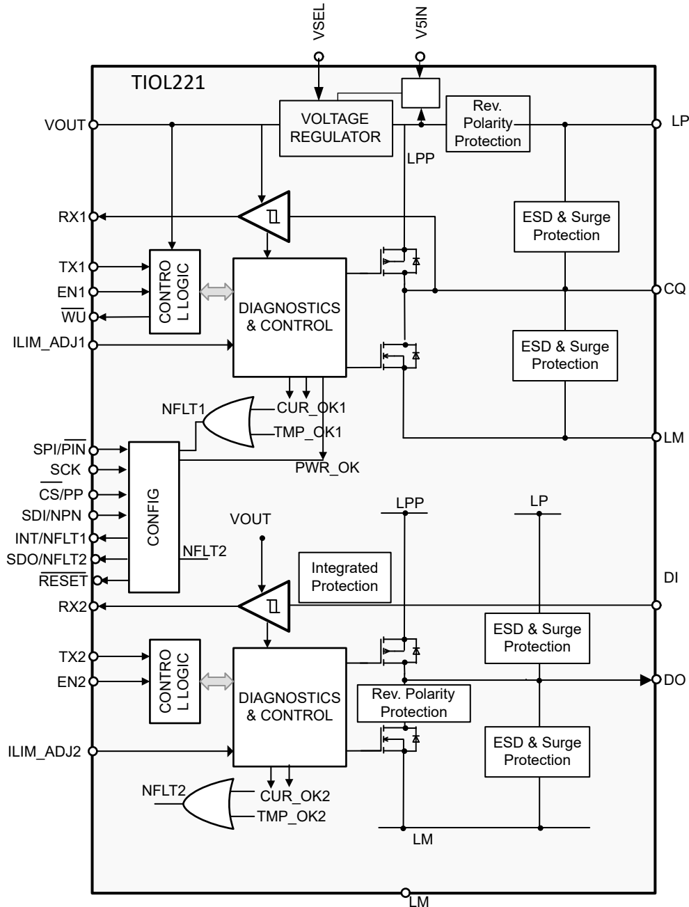
图 7-1. 方框图
