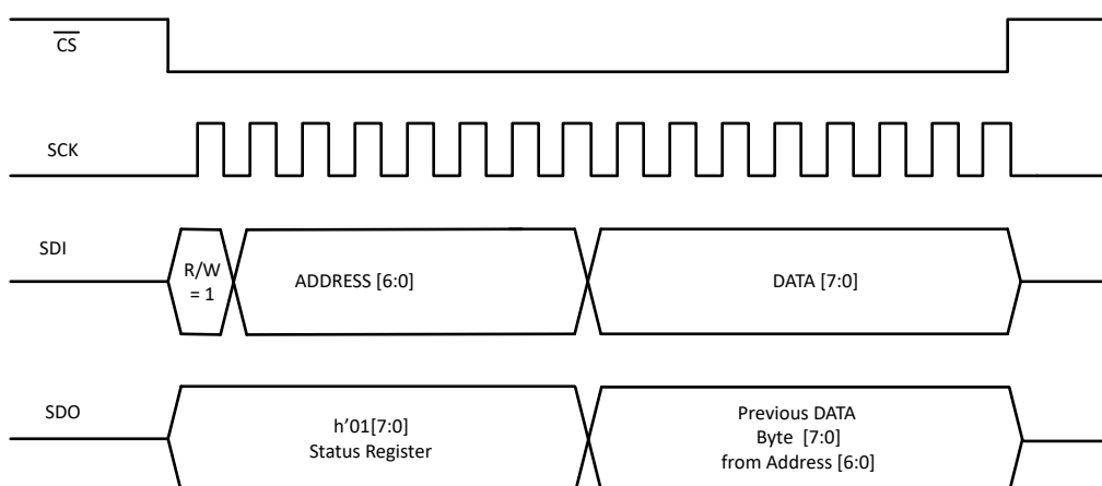
图 7-6. SPI 写入 (单字节)
