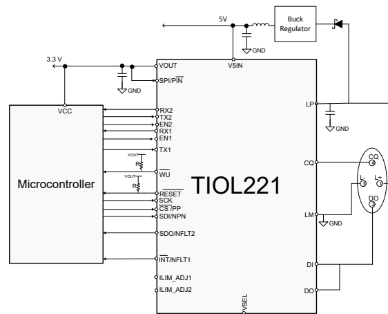
典型应用图
