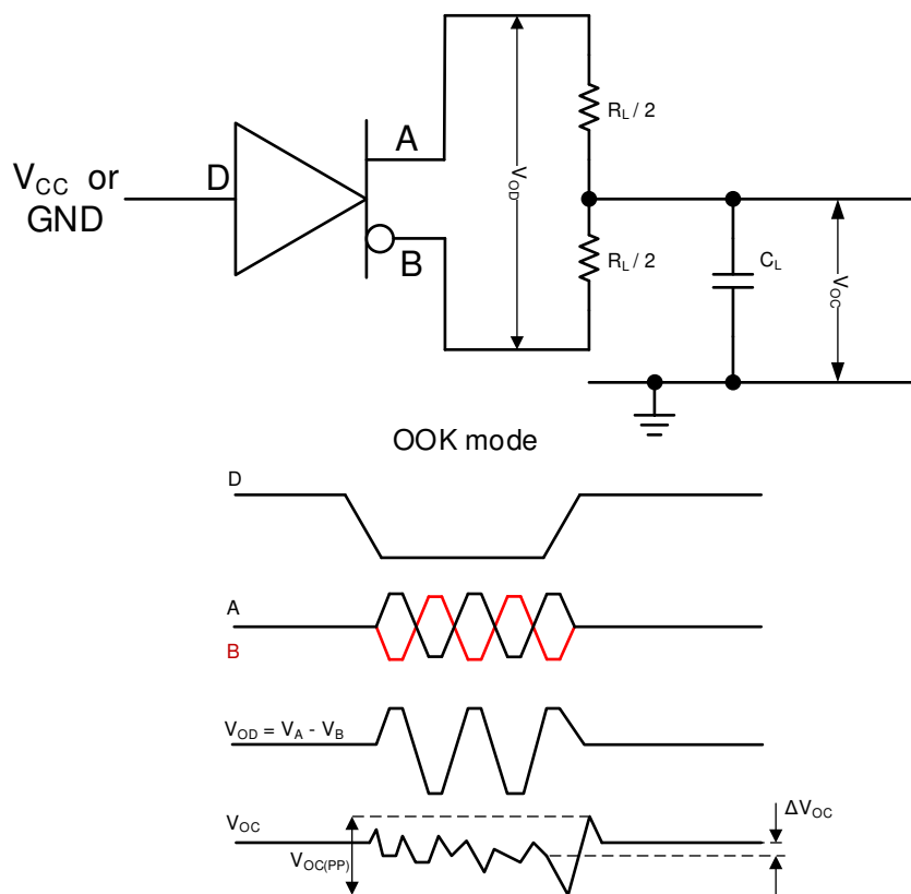
图 6-2. 驱动器差分 and 共模输出的测量
