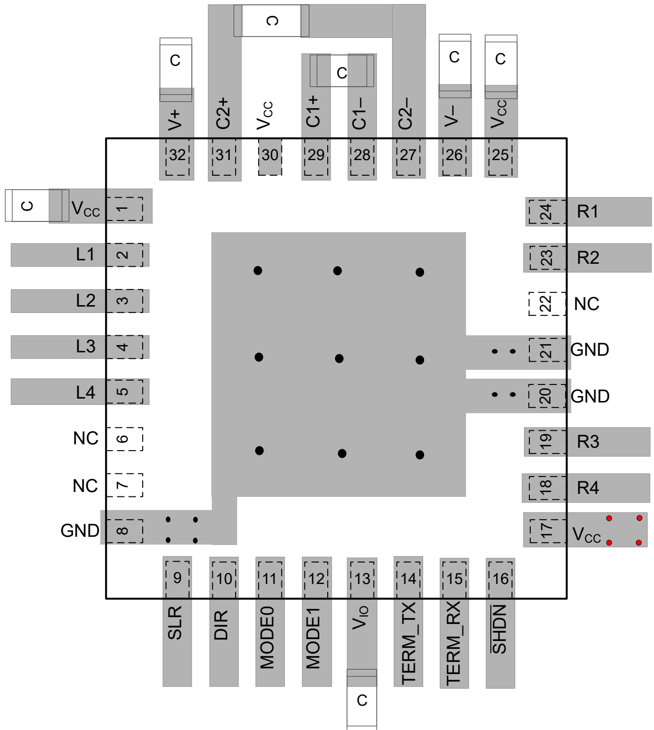
图 8-13. 布局示例
