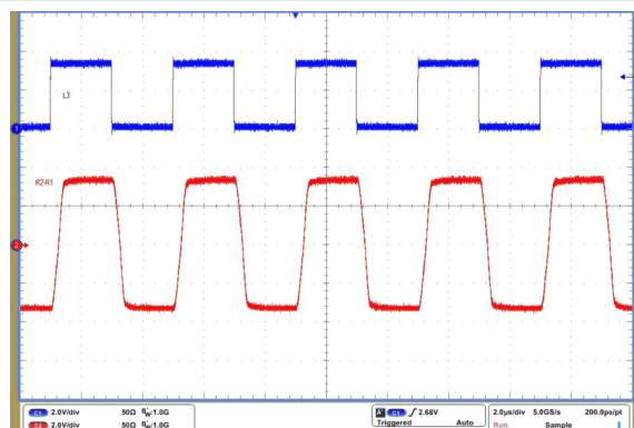
V_{CC} = 5V 总线负载 = 54\Omega || 50pF SLR = V_{IO} 500kbps 时的方波
