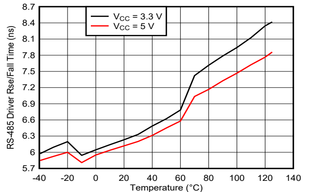
图 5-10. RS-485 20Mbps 驱动器上升时间或下降时间与温度间的关系
