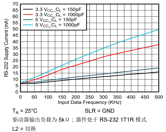
图 5-16. 1Mbps 模式下的 RS-232 电源电流与信号传输速率间的关系
