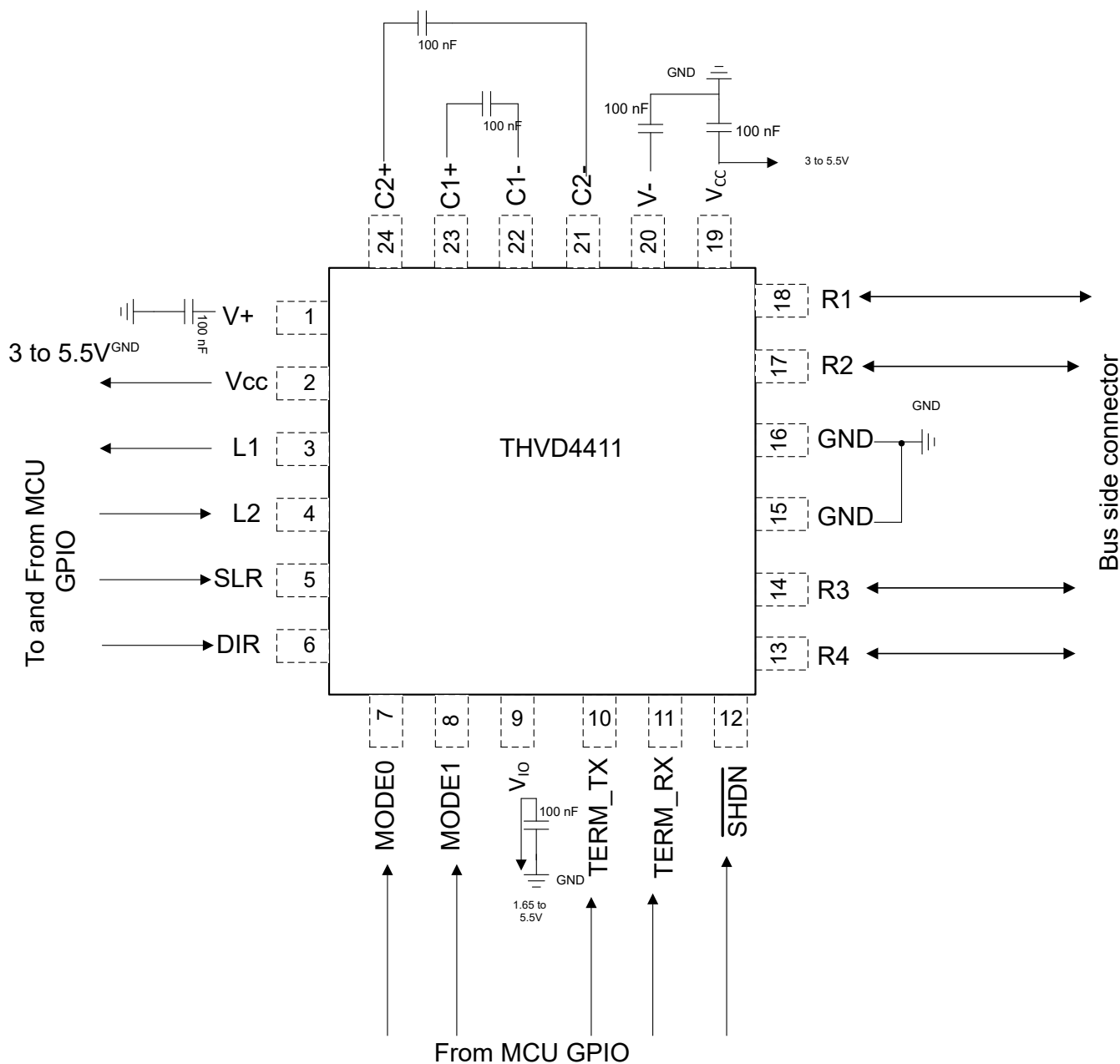
图 8-4. THVD4411 的典型应用图
