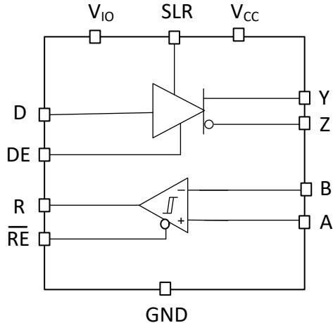
图 7-2. THVD2452V-EP 方框图
