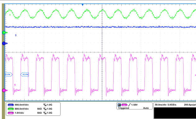
THVD2450V-EP 引脚 A 供电配置为 1.5V 直流偏置电压叠加 \pm 200\text{mV} 的动态范围
