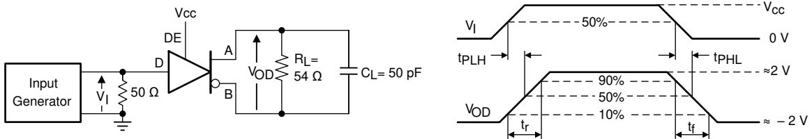
图 7-3. 驱动器差分输出上升和下降次数以及传播延迟的测量
