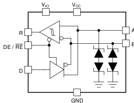
THVD14x9V 方框图
