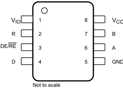
图 5-2. THVD1439V、THVD1449V，8 引脚 (SOIC)，顶视图
