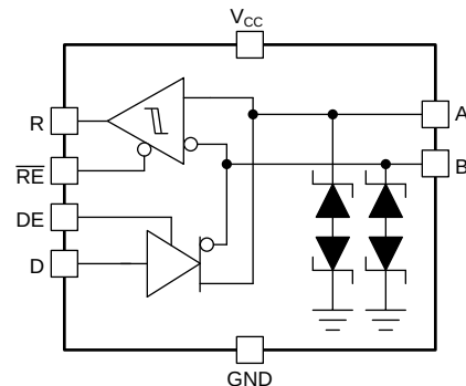
THVD1419 和 THVD1429 方框图
