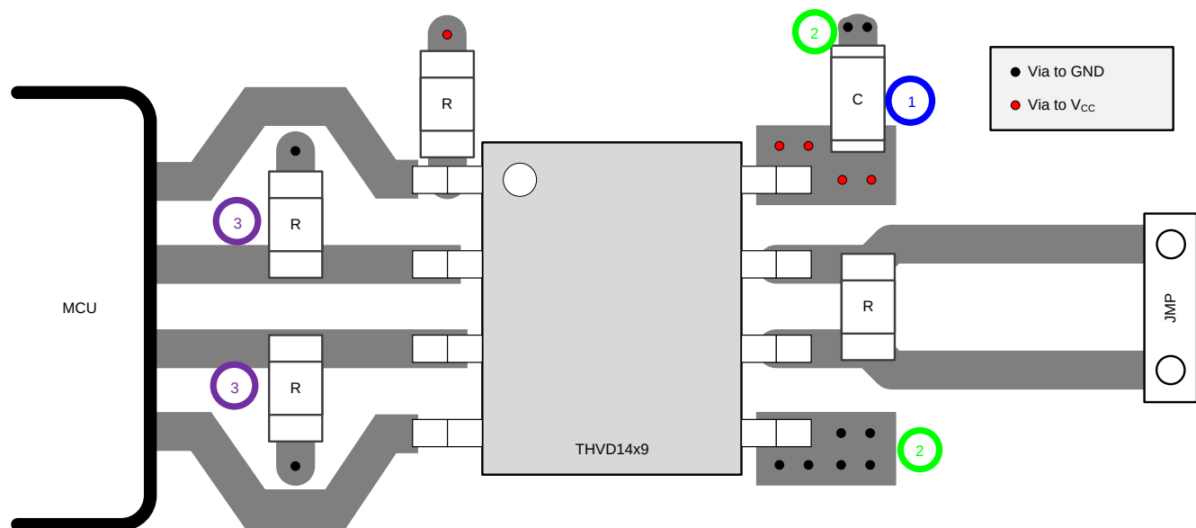
图 27. Half-Duplex Layout Example
