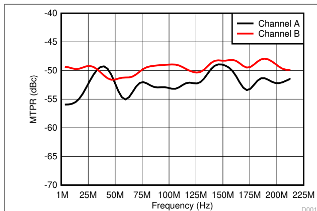
图 8-2. MTPR G.Fast 212-MHz
