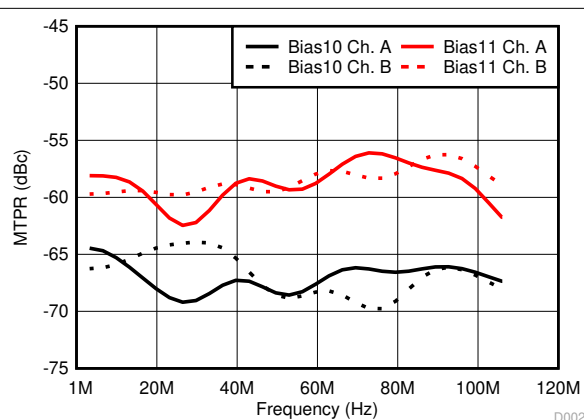
图 8-3. MTPR G.Fast 106-MHz
