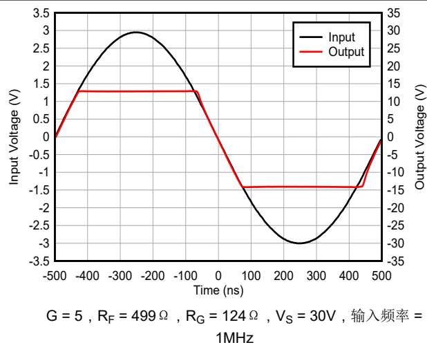
图 6-27. 过驱恢复
