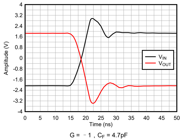
图 6-25. 趋稳时间
