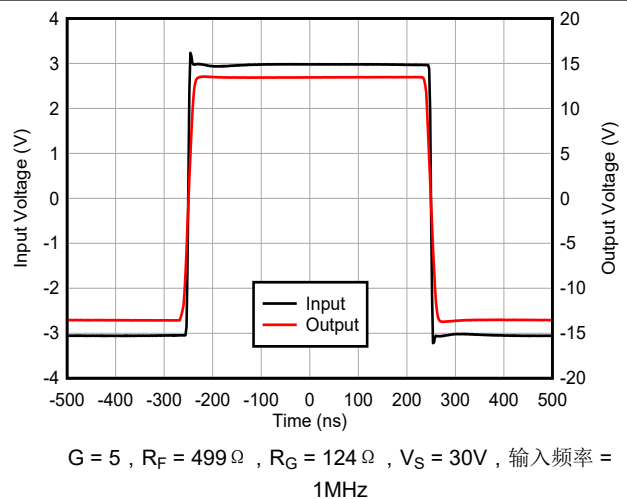
图 6-28. 过驱恢复
