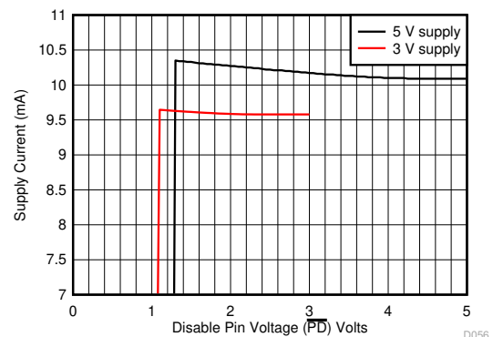
图 7-22. 电源电流与 \overline{PD} 电压之间的关系
