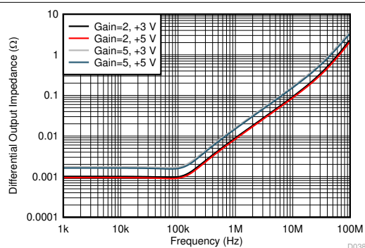
单端输入至差分输出，仿真差分输出阻抗，（闭环）增益为 2 和 5
