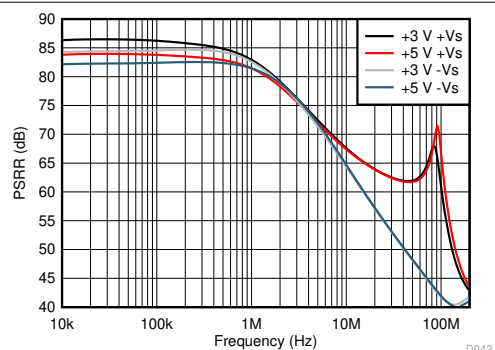
单端至差分，增益为 2 PSRR 仿真至差分输出
