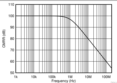
共模输入至差分输出，增益为 2 的仿真
