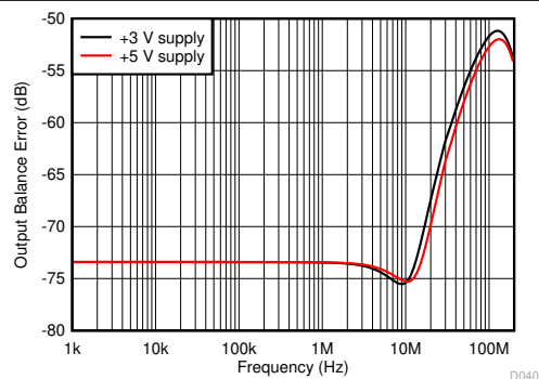
单端输入至差分输出，增益为 2，使用 1% 电阻器进行仿真，最坏情况失配
