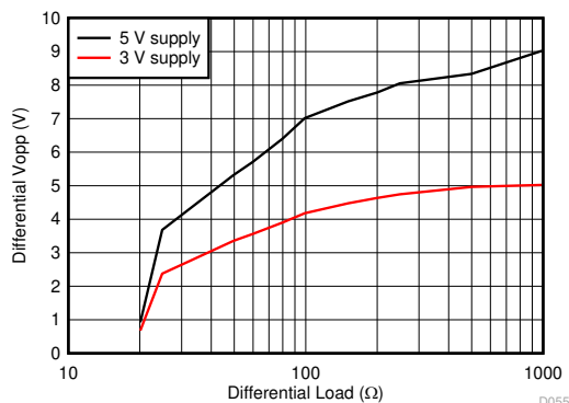
最大差分输出摆幅， 1/2 V_S 时的 V_{ocm}
