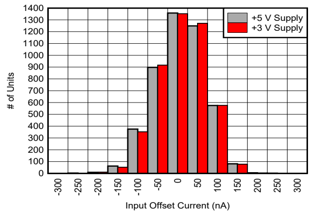
总共 4618 个单元，在 V_S = 5V 时： \mu = 16.7nA ， \sigma = 62.3nA
