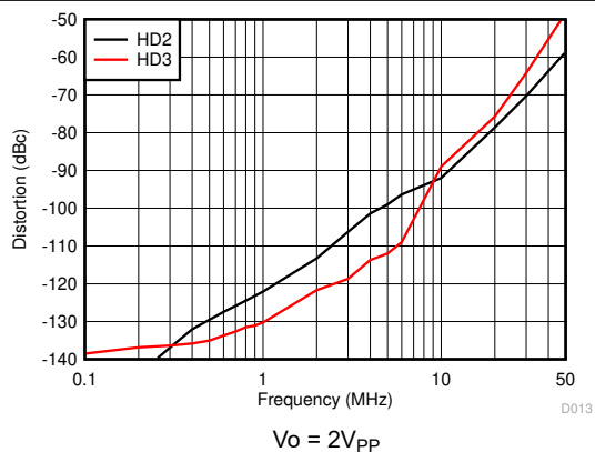
图 7-7. 谐波失真随频率变化的情况
