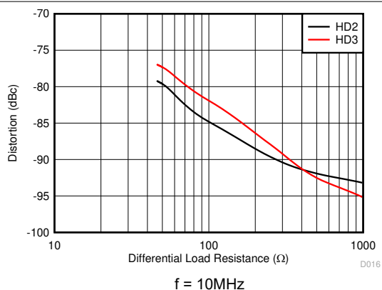
图 7-9. 谐波失真与 R_{load} 之间的关系
