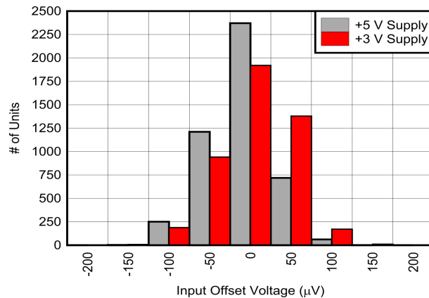
总共 4618 个单元，在 V_S = 5V 时： \mu = -35.1\mu V ， \sigma = 38.9\mu V
