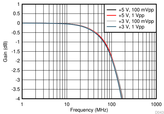
图 7-17. 共模，小信号和大信号响应 ( V_{ocm} 引脚驱动)
