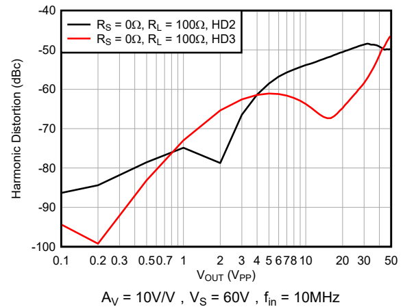
图 5-32. 谐波失真与输出电压间的关系
