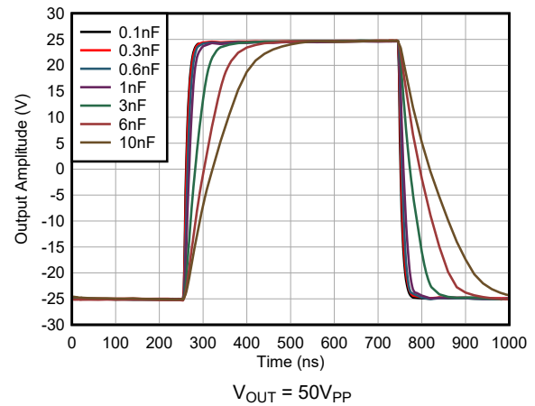
图 5-16. 大信号阶跃响应与电容负载间的关系
