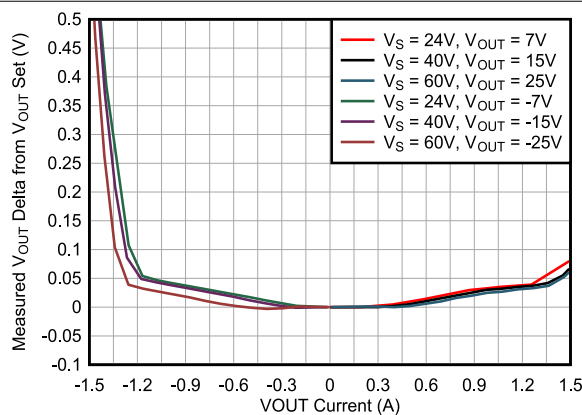
图 5-35. 输出余量与电源电压间的关系
