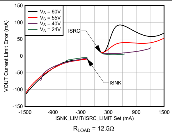
图 5-36. 输出电流限制与 ILIMIT 设置间的关系
