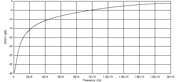
图 6-4. Input Differential Return Loss (SDD11)
