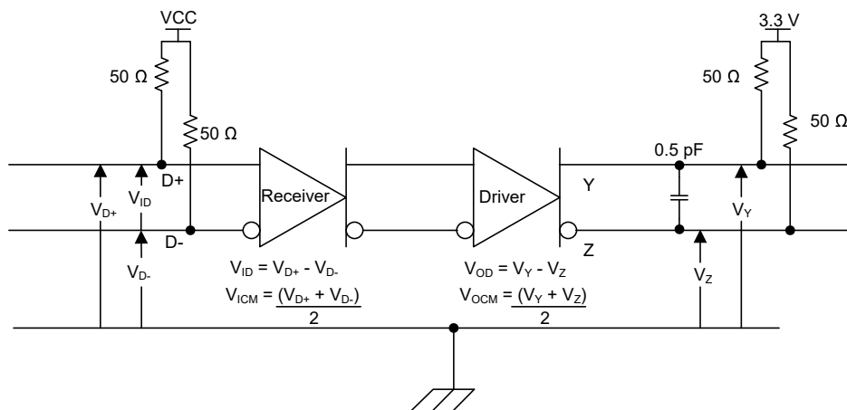
图 7-2. TMD5 Main Link Test Circuit
