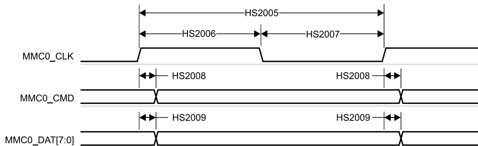
图 6-75. MMC0 - HS200 模式 - 发送模式
