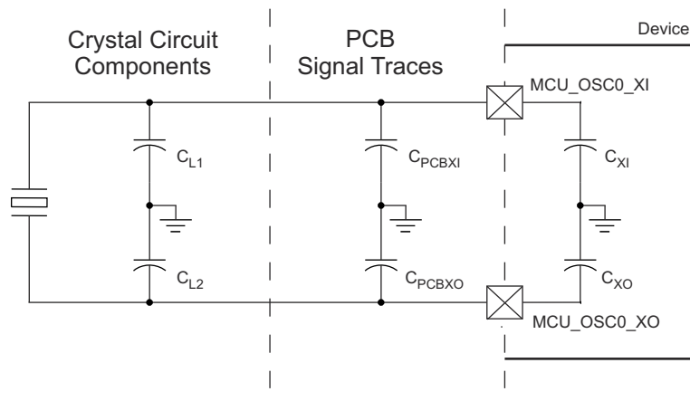
图 6-18. 负载电容
