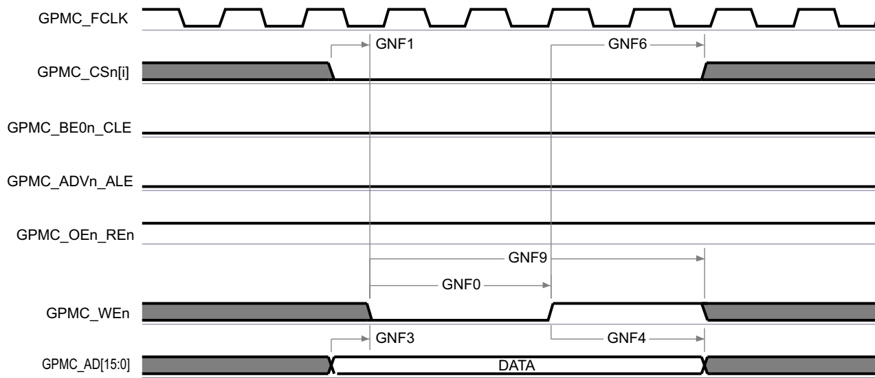
图 6-60. GPMC 和 NAND 闪存 - 数据读取周期
