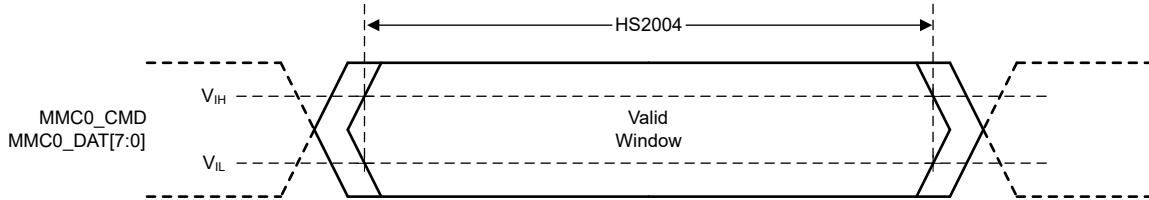
图 6-74. MMC0 - HS200 - 接收模式
