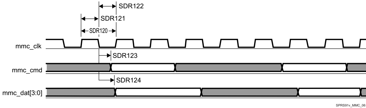
图 7-44. MMC/SD/SDIOj in - SDR12 - Transmitter Mode
