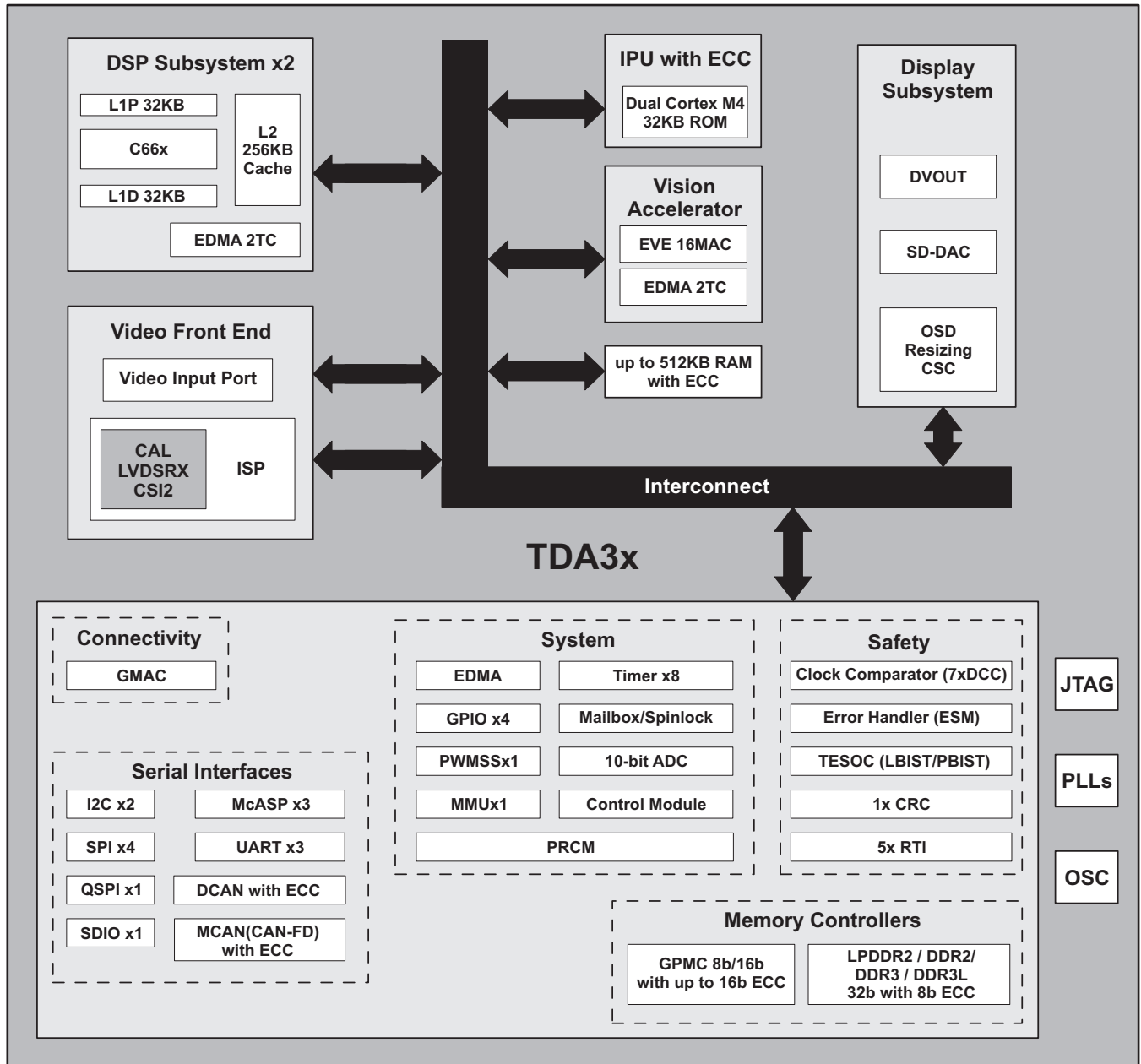
图 1-1. TDA3x 框图
