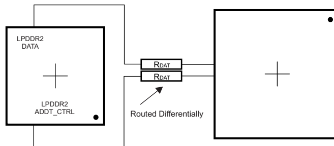
图 8-28. DQ[x] Topology
