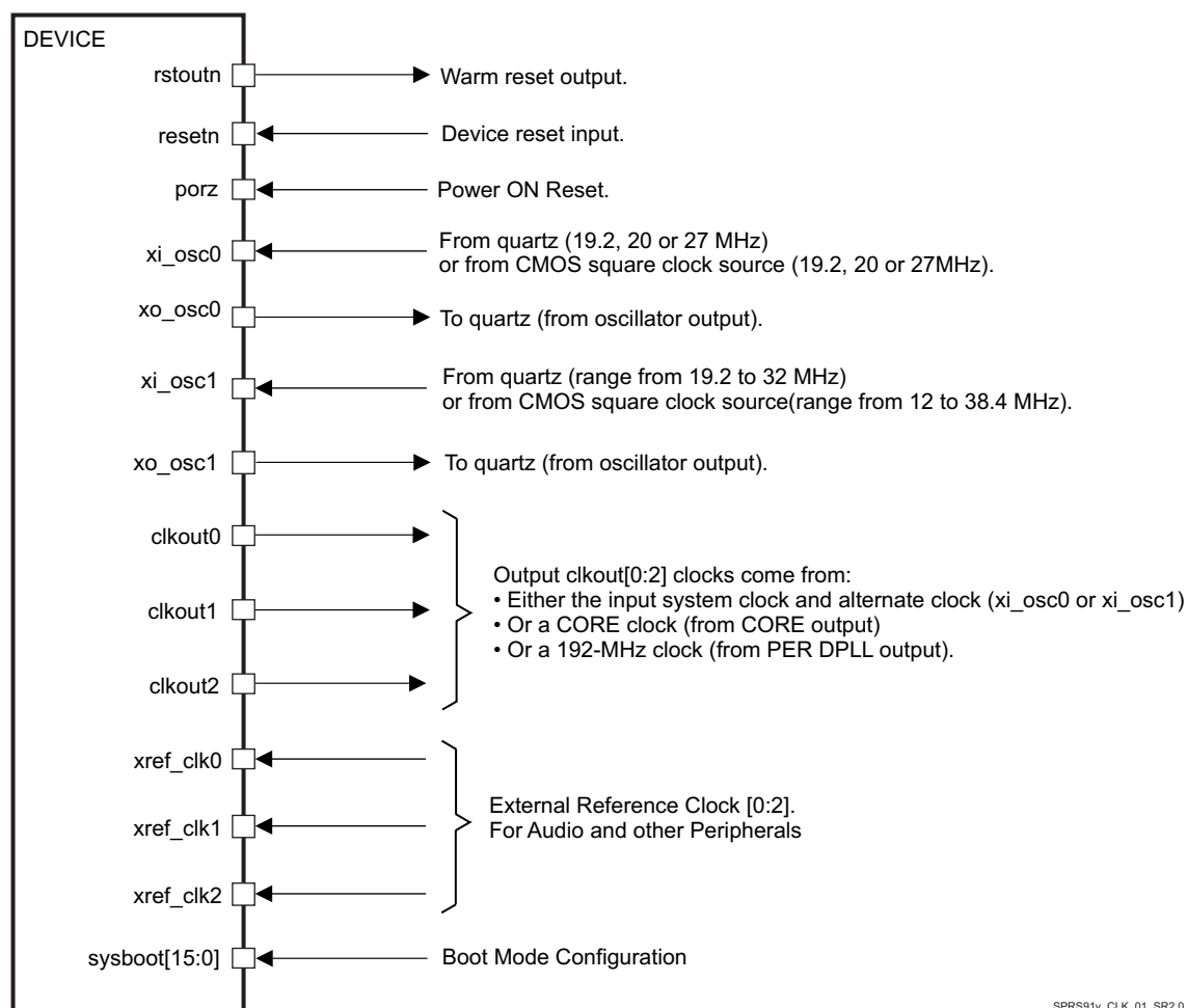
图 6-1. Clock Interface
