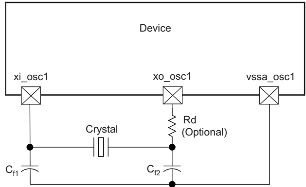
图 6-6. Crystal Implementation
