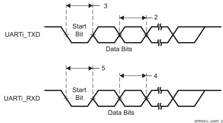
图 7-25. UART Timing
