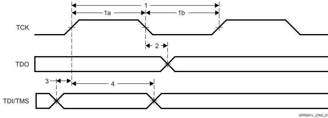
图 7-47. JTAG Timing
