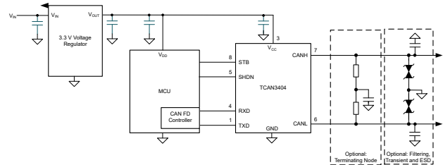
简化原理图
