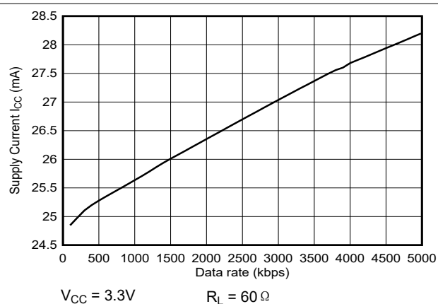
图 6-6. I_{CC} vs Data Rate
