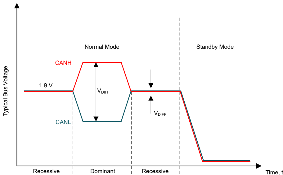
图 8-2. Bus States
