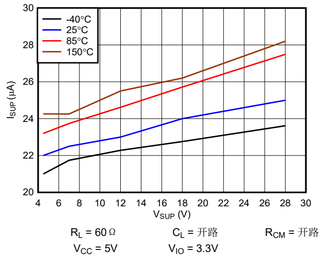
图 5-3. 睡眠模式下的 I_{SUP} 与 V_{SUP} 和温度间的关系
