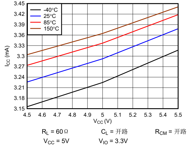
图 5-2. 隐性 I_{CC} 与 V_{CC} 和温度间的关系
