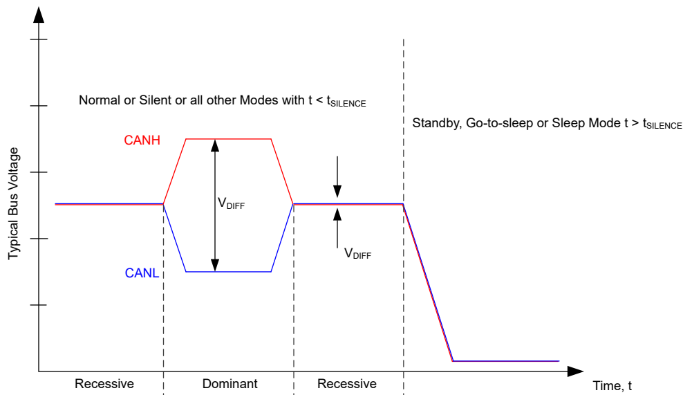
图 7-12. 总线状态
