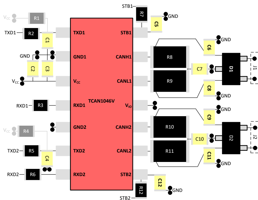
图 11-1. Example Layout
