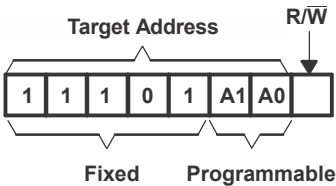
图 7-7. TCAL9539R 地址
